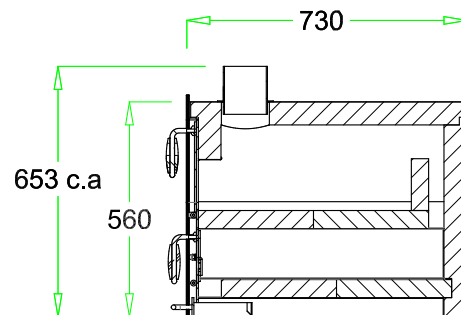
SEZIONE A-A
